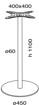
Punto 433 bar table base
