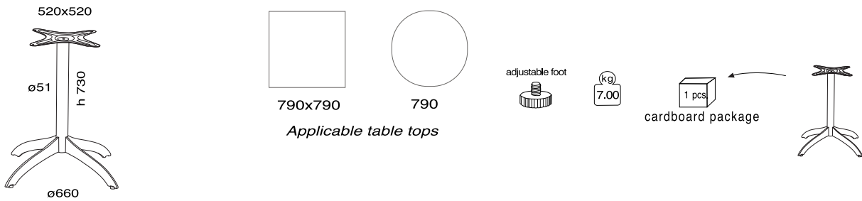
Arya 330 Table base
