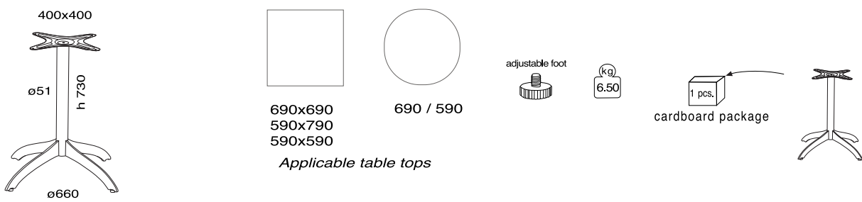
Arya 331 Table base
