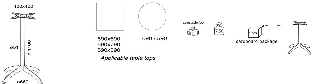
Arya 332 Bar Table base
