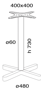
Kross 371 side table base
