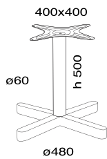
Kross 371 side table base
