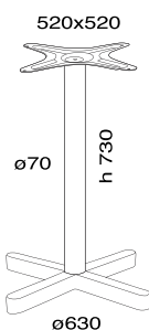
Kross 372 table base
